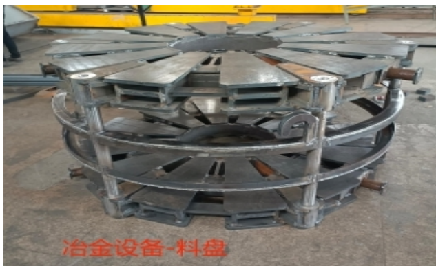
料盘，用于铜带热处理
