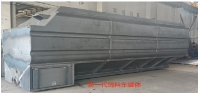
Y41D罐体，容积：41m 3 ，卸料方式：绞龙 材质：碳钢，用途：饲料运输
